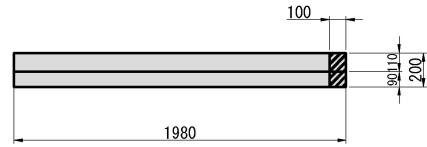
側面図
