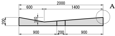
断面図
